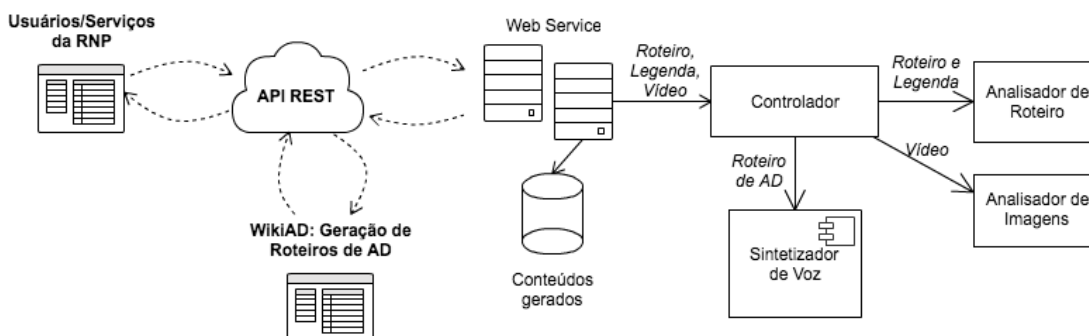
Figura 1. Arquitetura do Serviço Piloto (Audiodescrição@RNP)
